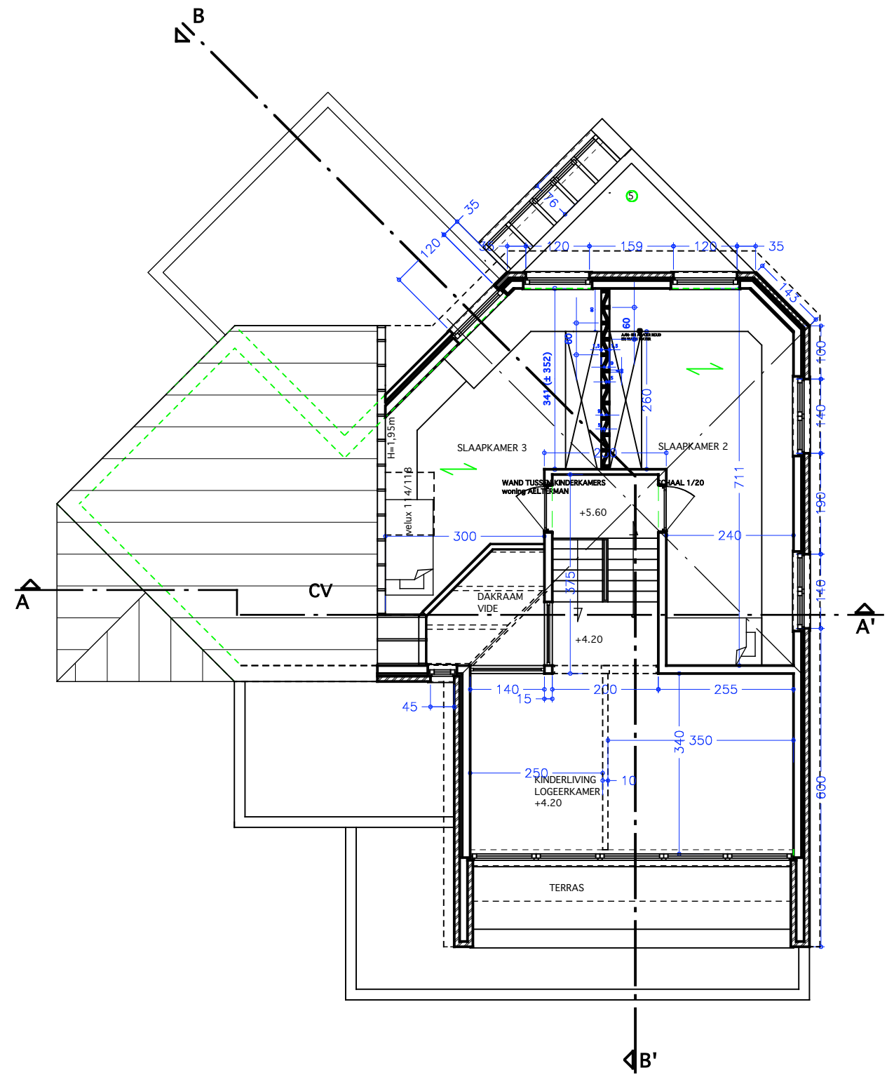
VERDIEPINGSPLAN NIV. 4.20 NIV. 5.60
