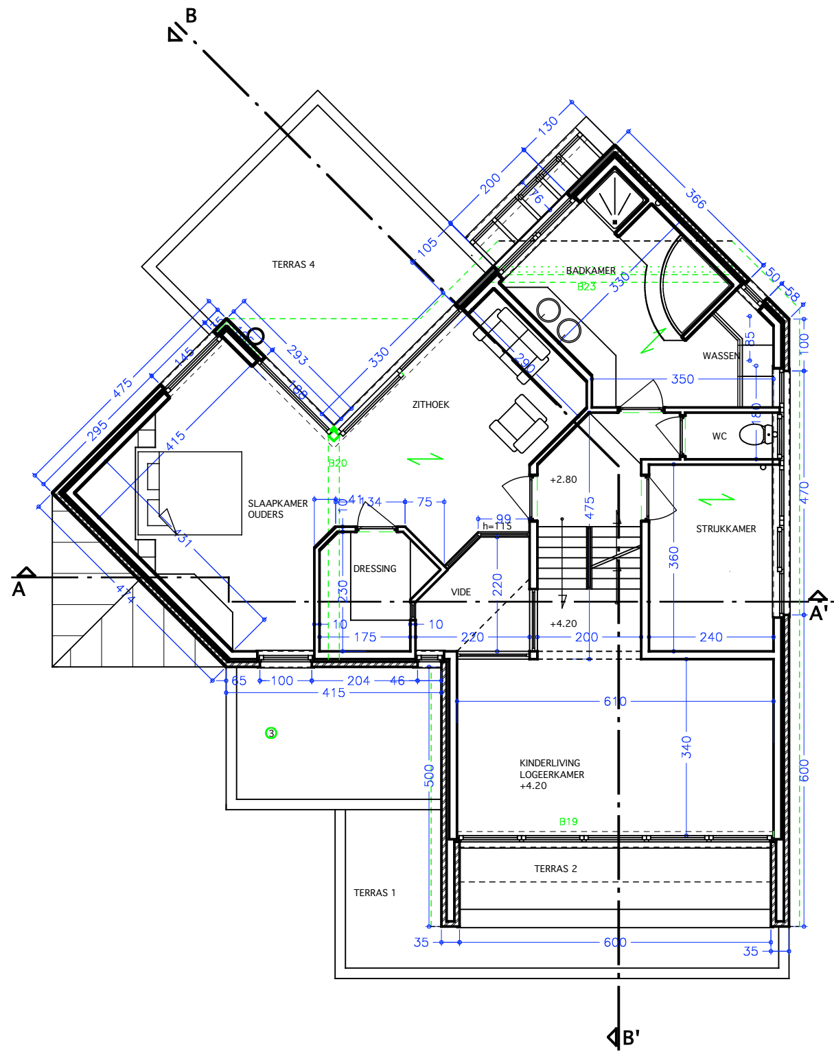
VERDIEPINGSPLAN NIV. 2.80 NIV. 4.20
